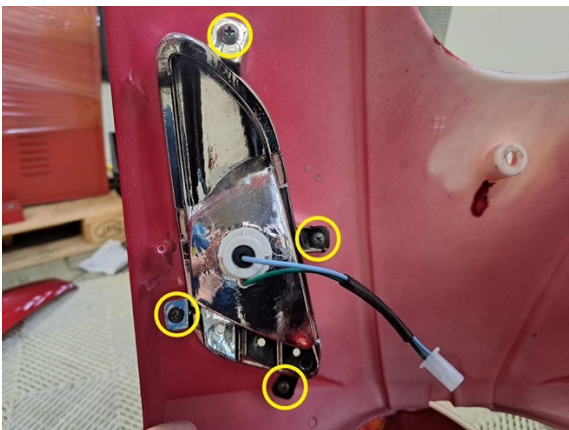
Irrota oikean etuvilkun kiinnitysruuvit. (ristipäämeisseli ph2).
