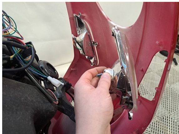
Ota oikeavilkku pois.
